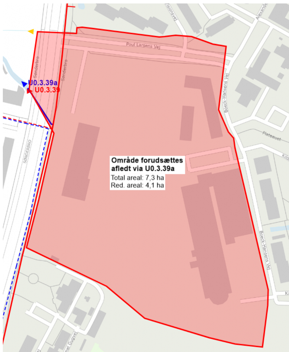
Figur 1: Situationsplan over område med afledning til U0.3.39a
