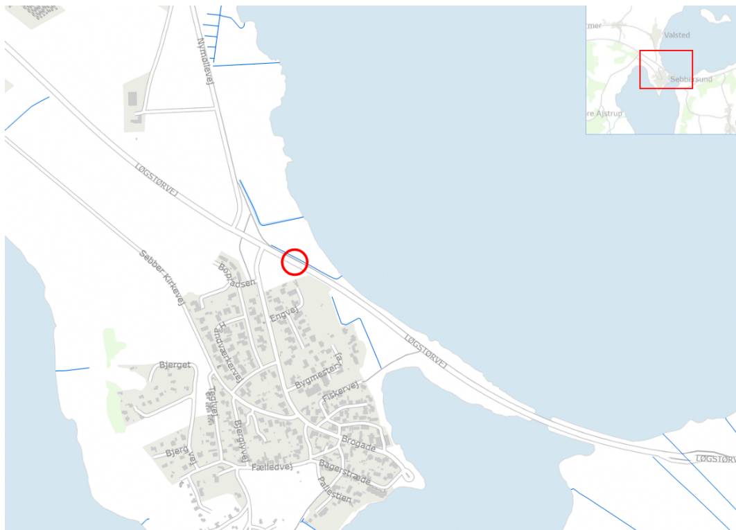
Figur 1 Omlægning af privat vandløb i forbindelse med etablering af busstoppested ved Sebbersund. Placeringen er markeret med en rød cirkel - vejnr. 800714 fra kmt 2/0639 til kmt 2/0726.
