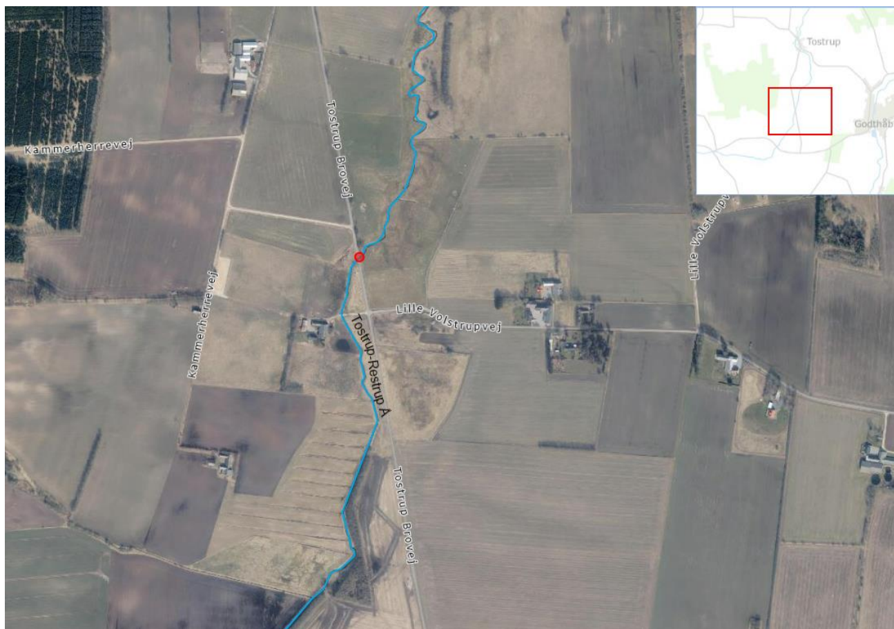
Figur 1: Placering af krydsning af Tostrup-Restrup Å med fibernet i station 958 på matr.nr. 7000e/7000l. Vandløb er markeret med blå streg og krydsning er markeret med rød cirkel.
