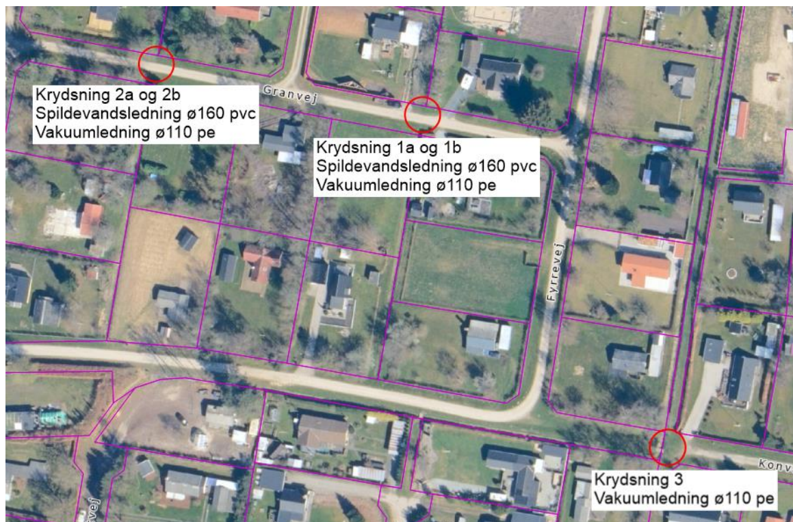
Figur 1 Oversigtskort over krydsningerne af de tre private grøfter på matr.nr. 20c og 21a, Egense By, Mou. Krydsningerne er markeret med en rød cirkel.
